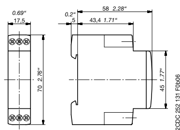
Устройства СТ-D с 1 переключающим контактом или 2 НО контактами
