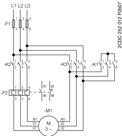
Схема цепи питания
